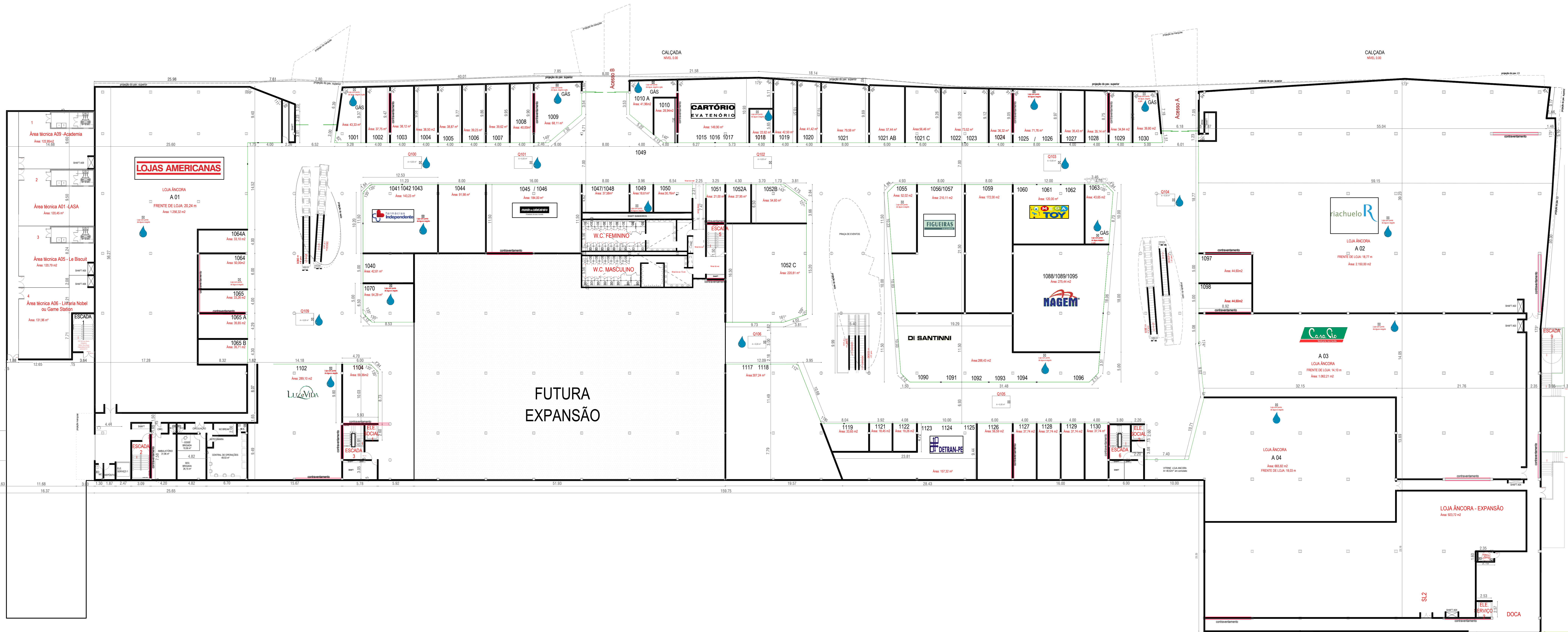
PLANTA BAIXA PAVIMENTO L1 ESCALA 1/200
