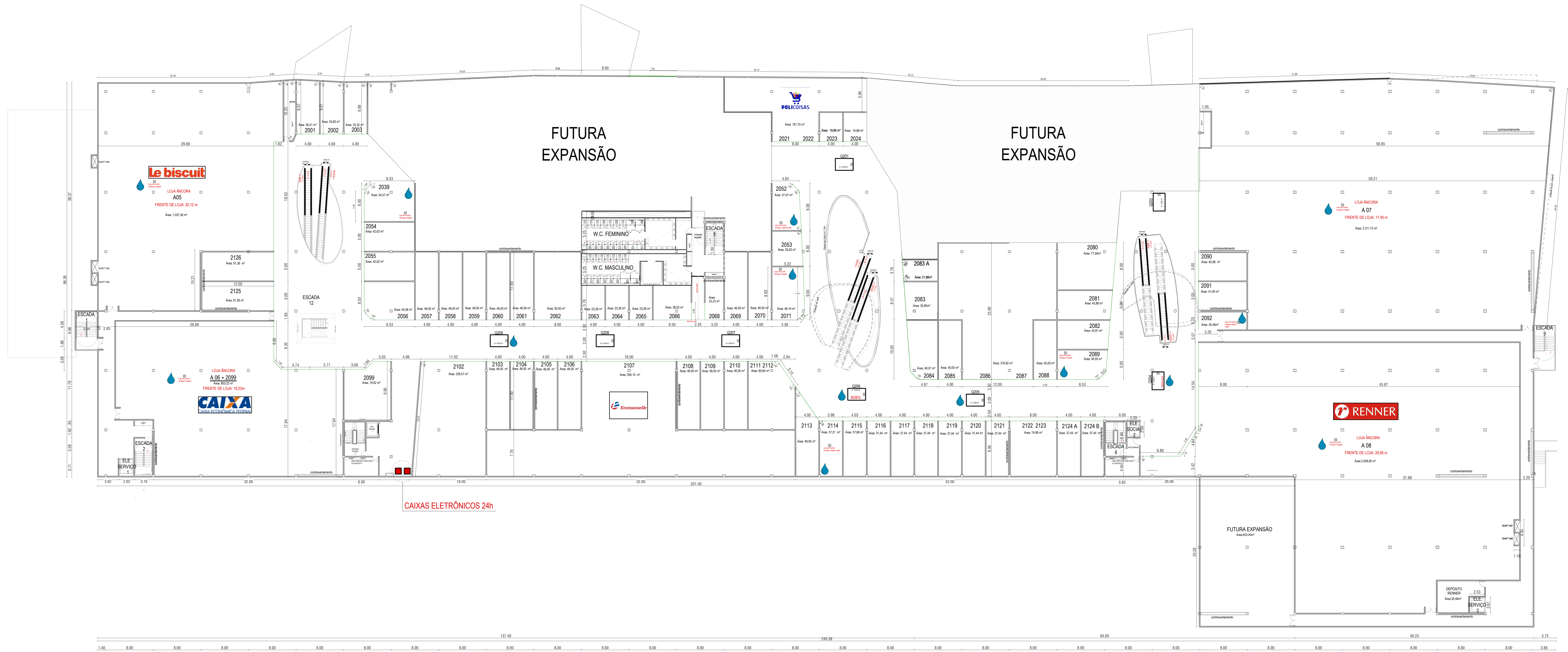
PLANTA BAIXA PAVIMENTO L2 ESCALA 1/200
